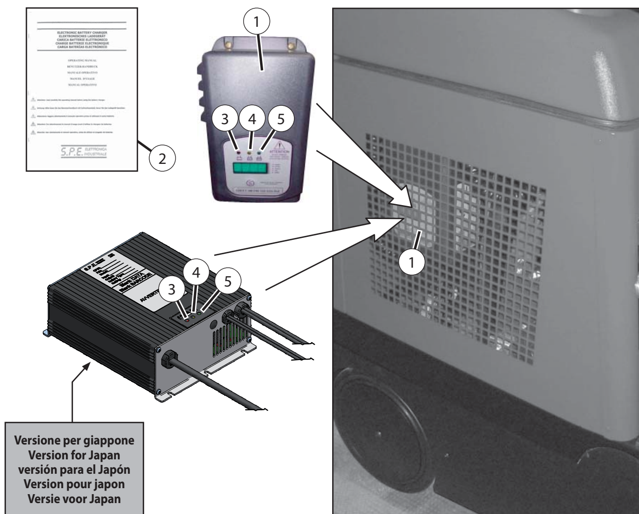
FIG.13A
